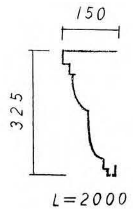
Ante-MS-F 325-150(**FRP)
