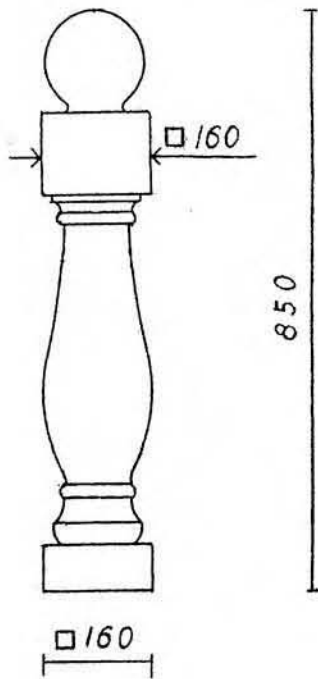
Ante-PS 00 (**FRP)
