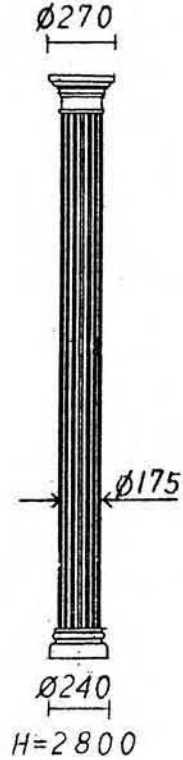
Ante-C-PS-F 175(**FRP)
