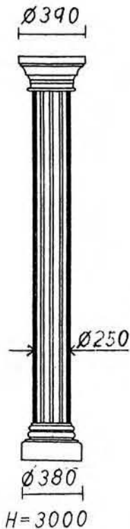
Ante-C-PS-F 250(**FRP)
