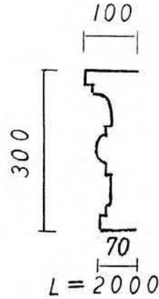
Ante-MS-F 300-100(**FRP)
