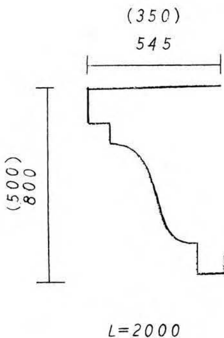
Ante-MS-F 800-545 / 500-350 (**FRP)
