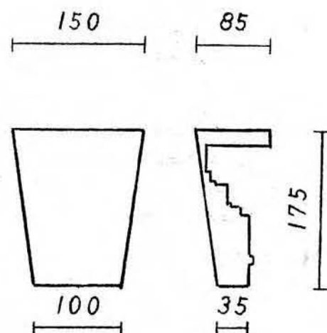
Ante-KSS 150-72
