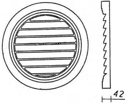
Ante-RLS 450
