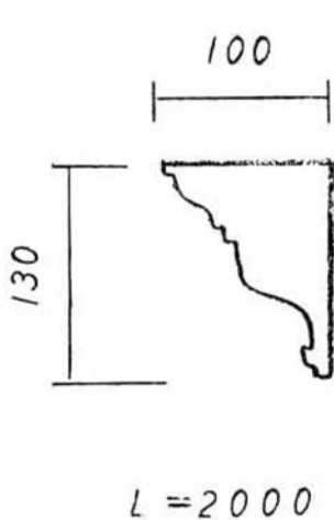
Ante-MS-P 130-100(**PUF)
