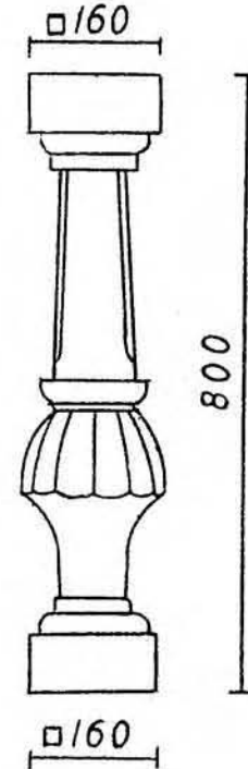
Ante-BAS 03 (**FRP)
