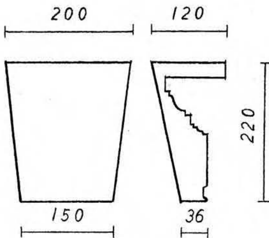
Ante-KSS 200-95
