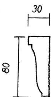
Ante-MS-P 80-30(**PUF)
