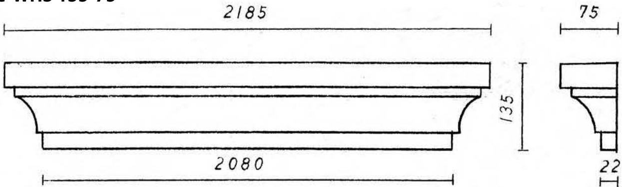
Ante-WHS 135-75
