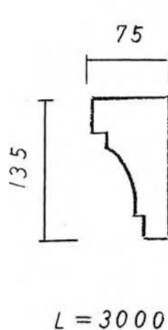
Ante-MS-P 135-75(**PUF)
