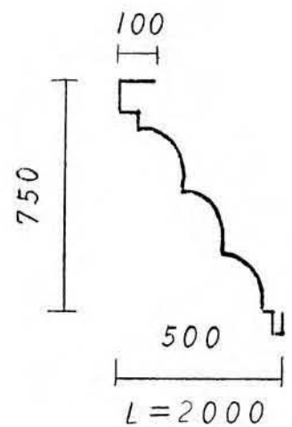
Ante-MS-F 750-500(**FRP)
