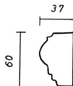
Ante-MS-P 60-37(**PUF)
