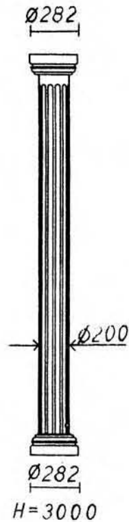
Ante-C-PS-F 200(**FRP)
