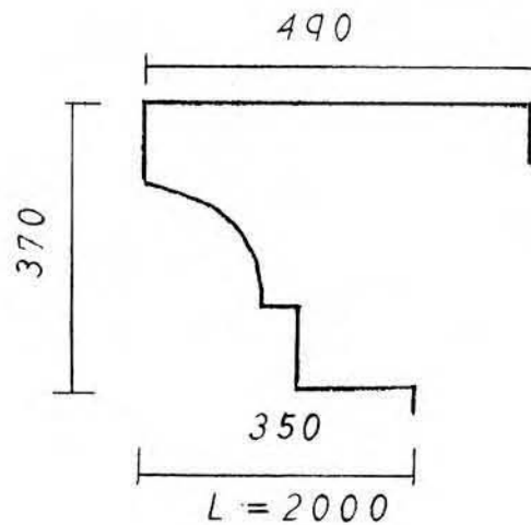
Ante-MS-F 370-350(**FRP)
