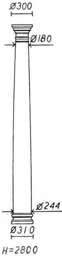
Ante-C-PS-F 250(**FRP)
