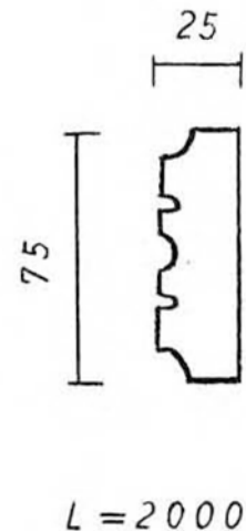
Ante-MS-P 75-25(**PUF)
