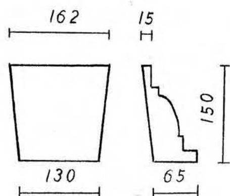
Ante-KSS 135-75 B
