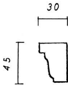
Ante-MS-P 45-30(**PUF)
