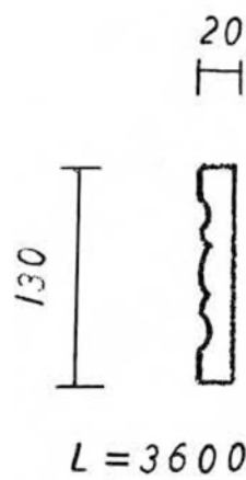
Ante-MS-P 130-20(**PUF)
