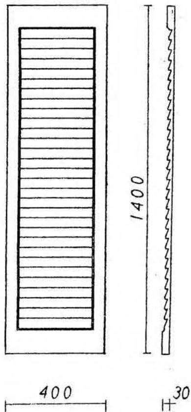
Ante-PLS 1400-400
