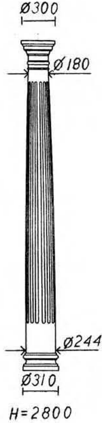
Ante-C-PS-F 200(**FRP)
