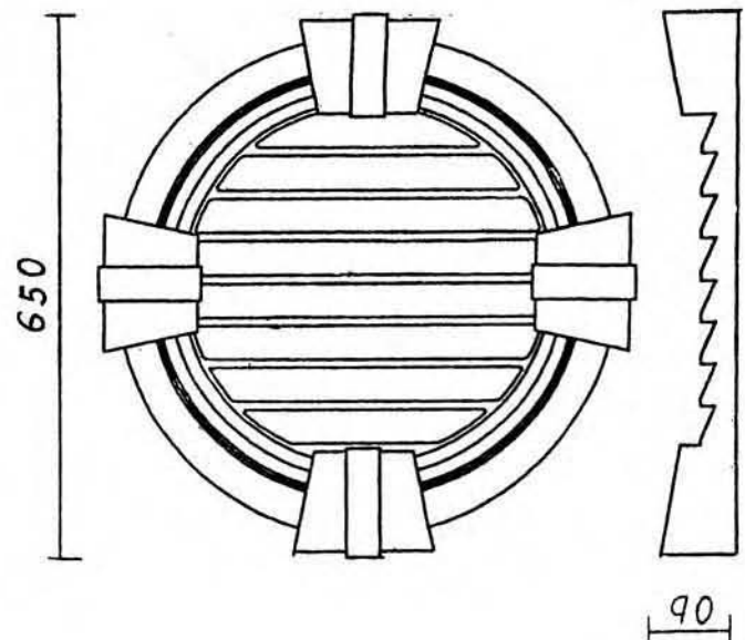
Ante-RLS 600 K
