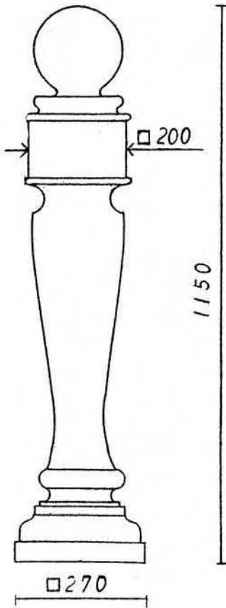
Ante-PS 02 (**FRP)
