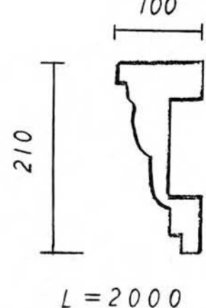
Ante-MS-P 210-100(**PUF)
