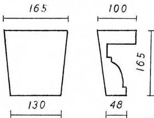
Ante-KSS 135-75 A
