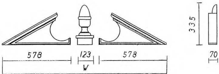
Ante-PS 1284
