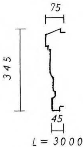
Ante-MS-F 345-75(**FRP)
