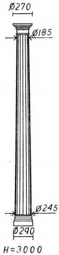
Ante-E-PS-F 003(**FRP)
