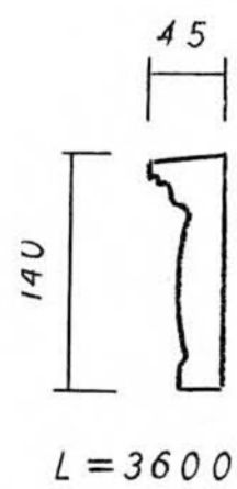
Ante-MS-P 140-45(**PUF)
