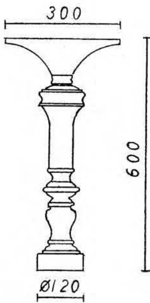
Ante-BAS 01 (**FRP)
