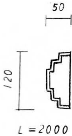
Ante-MS-P 120-50(**PUF)
